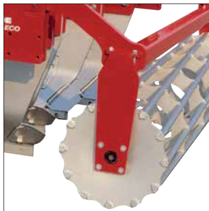
Kongskilde Paragrubber ECO 3000 csőhengerrel.
