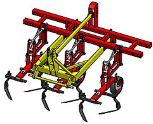
FRONT FÜGGESZTÉS KULTIVÁTOR
