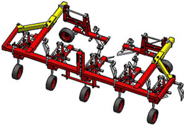
HÁTRA CSUKODÓ KULTIVÁTOR
